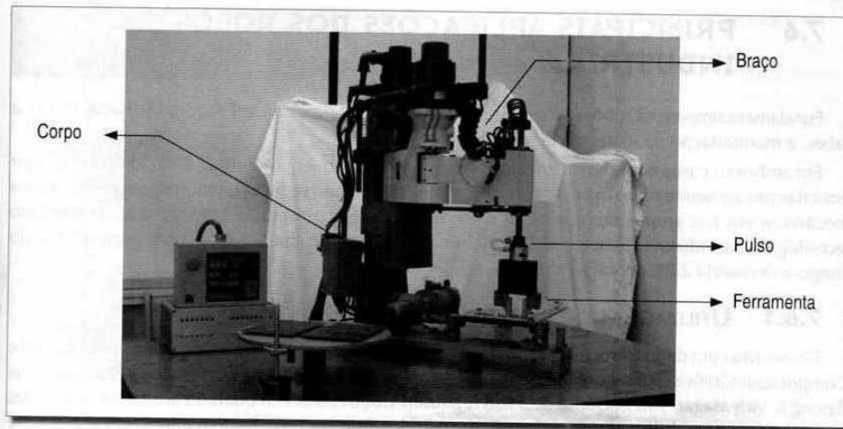
Figura 7.2 Estrutura de um robô em analogia com o ser humano.
